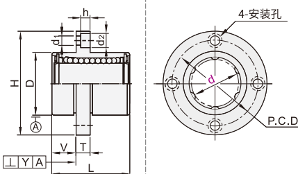
圆法兰型 ELU01E/02E
