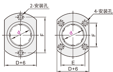
对边法兰型 ELU31E/32E
