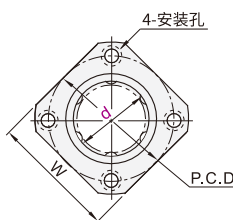
方法兰型 ELU21E/22E
