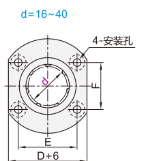
对边法兰型 ELL71/72
