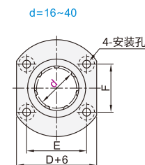
对边法兰型 ELL31/32
