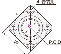
方法兰型 ELL61/62
