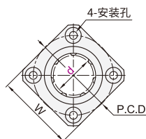
方法兰型 ELT21/22
