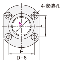
对边法兰型 ELT31/32
