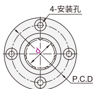
圆法兰型 ELT01/02
