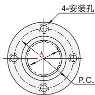
圆法兰型
