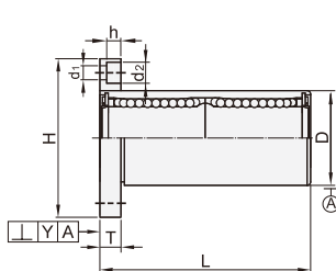
■单衬型
