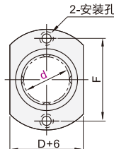
对边法兰型
