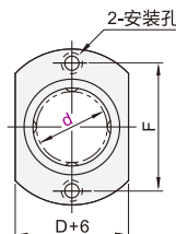
对边法兰型
