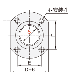
对边法兰型 ELZ31MX ELZ32MX
