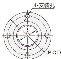
圆法兰型 ELZ01MX ELZ02MX
