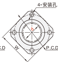
方法兰型 ELW21MX ELW22MX
