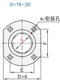
对边法兰型 ELW31MX ELW32MX
