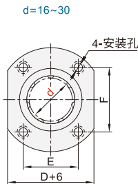
对边法兰型 ELU31MX ELU32MX
