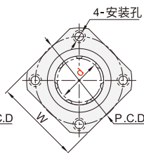
方法兰型 ELU21MX ELU22MX
