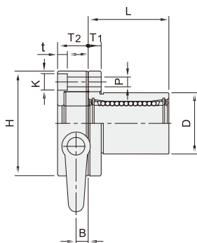
右把手 单衬型
