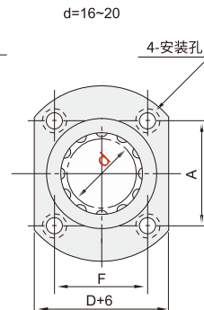
两面切割法兰型
