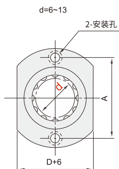
两面切割法兰型
