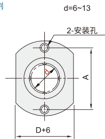
两面切割法兰型
