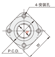
方法兰型
