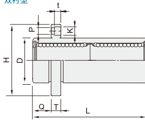
双衬型
