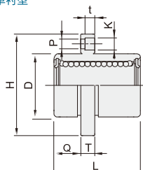
单衬型
