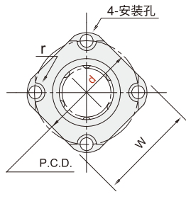
方法兰型
