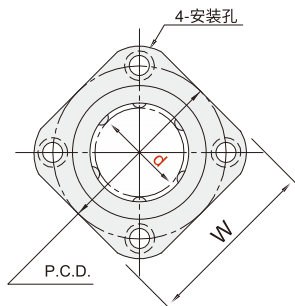
方法兰型
