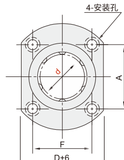
两面切割/法兰型
