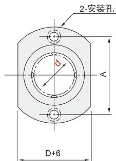
两面切割/法兰型
