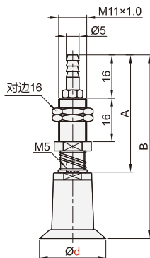
HDSR43 直立配管弹簧型
