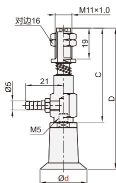
HDSR44 侧端配管弹簧型
