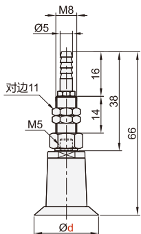
HDSR41 直立配管型
