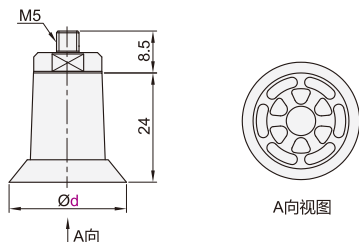
HDSR43 直立配管弹簧型
