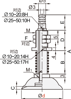
盘径 \varnothing 15-50
