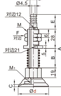
盘径 \varnothing 60-95
