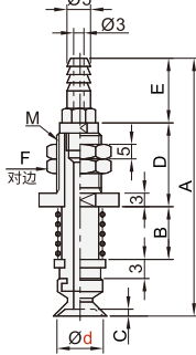
盘径 \varnothing 10
