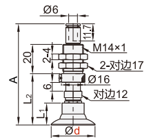
弹簧式直接安装型 HDSL67/68
