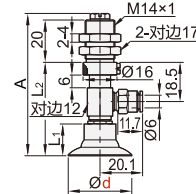
弹簧式侧面真空端口 HDSL65/66
