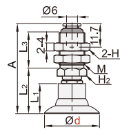
固定式顶部真空端口 HDSL61/62
