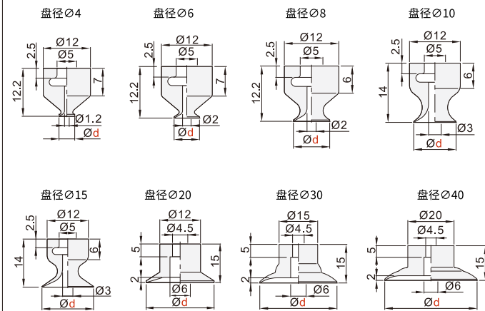
弹簧式侧面真空端口 HDSL65/66
