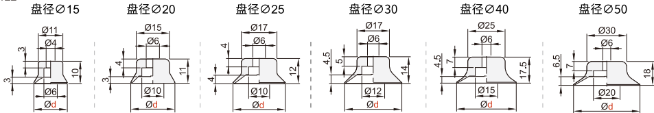
固定式顶部真空端口 HDSK31/32
