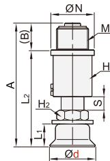
弹簧式直接安装型 HDSK45/46
