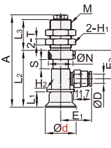
弹簧式侧面真空端口 HDSK43/44/
