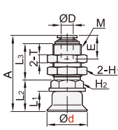
固定式顶部真空端口 HDSK31/32
