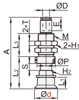
弹簧式顶部真空端口 HDSK41/42
