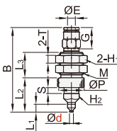
弹簧式顶部真空端口 HDSK21/22/23
