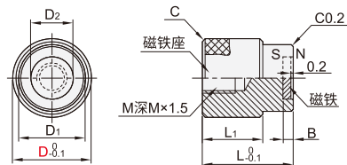
偏心薄型 GYLM71
