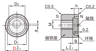
偏心薄型 GYLM71
