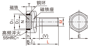
短头内六角孔型 GYLL36
