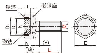
短头型 GYLL31
