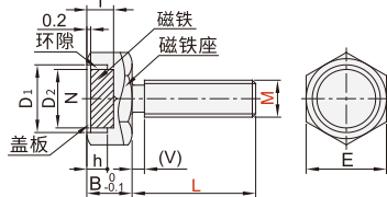
带盖型 GYLL21
