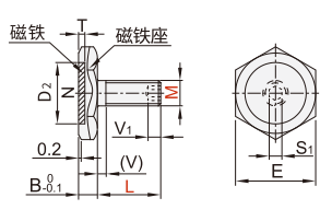
超薄短头内六角孔型 GYLL46
