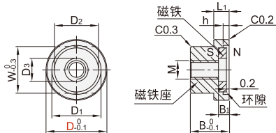
内螺纹调整型 YLK11
