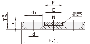
沉孔型 GYLG01/06
