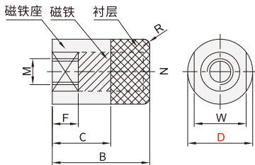
内螺纹型 YMQ21
