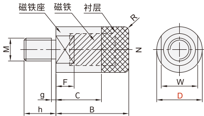
外螺纹型 YMQ11/12
