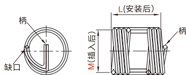
标准型 PLM01 PLM11
