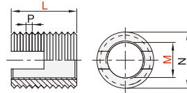
自攻开槽型 PLM31 PLM41
