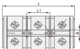
TC大电流端子排 JOTC91
