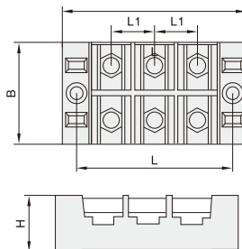
TB固定式端子排 JOTD41
