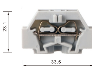
262-301-307 厚度:7mm
