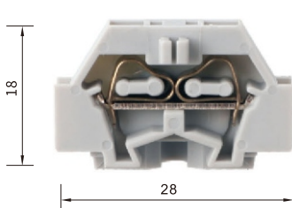
261-301-307 厚度:6mm
