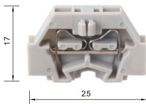
260-301-307 厚度:5mm
