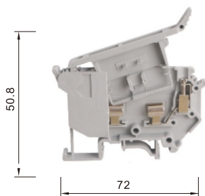
UK5-HESI保险端子 厚度:8.2mm
