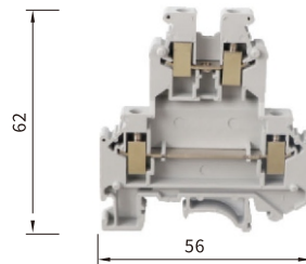
UKK3PV(上下联通) 厚度:5.2mm
