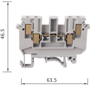
UDK4 厚度:6.2mm
