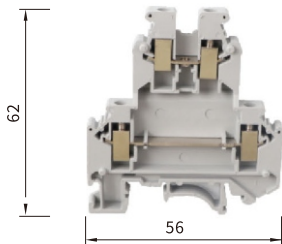
UKK3 厚度:5.2mm
