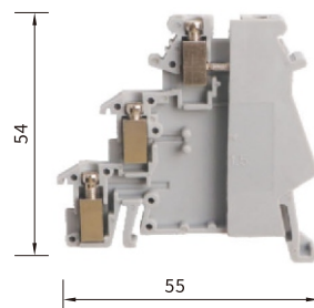
IK1.5 三层传感器端子 厚度:6.2mm
