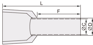
VE冷压端子 JDZB31
