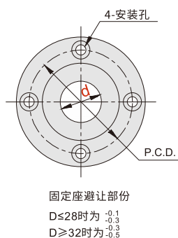
圆法兰型
