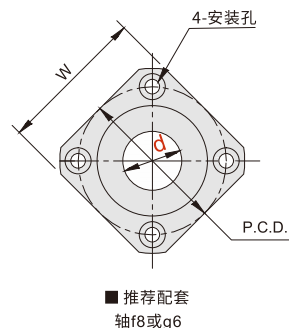
方法兰型
