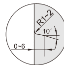
A部详图
