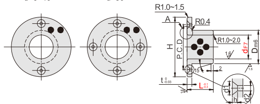
FDK02 锥孔型
