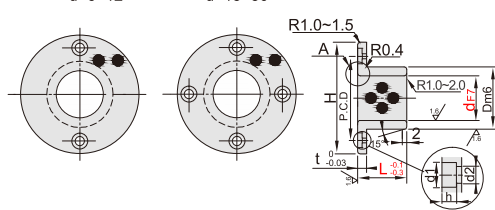
FDK03 沉孔型
