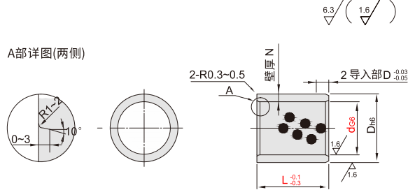
FCH02 薄壁型内径G6外径h6型
