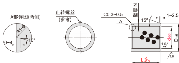
FCH01 标准型内径G6外径m6型
