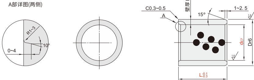
FCG02 薄壁型同径E7外径r6型
