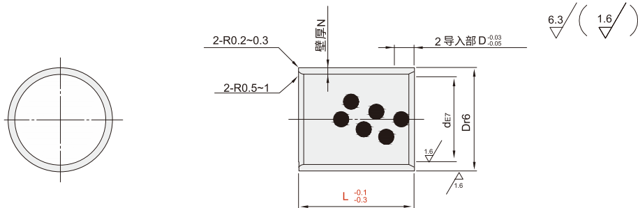
FCG02 薄壁型同径E7外径r6型
