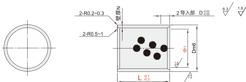
FCE02 薄壁型同径F7外径m6型
