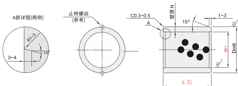
FCE01 标准型同径F7外径m6型
