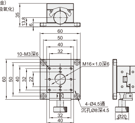
XY轴 DWE01-40 (铝合金) (黑色阳极氧化)
