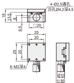
X轴 DWD01-25 (铜合金) (黑色氟树脂)
