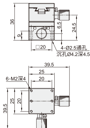
XY轴 DWE01-25 (铝合金) (黑色阳极氧化)
