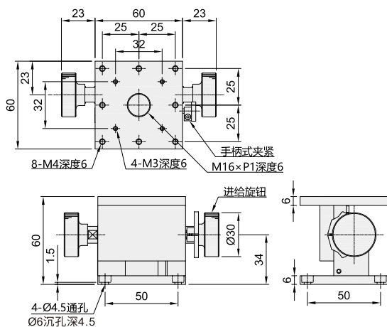
DXF31-60(铝合金)(黑色阳极氧化)
