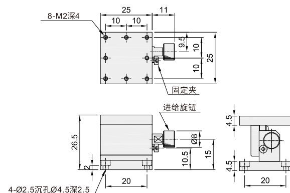
DXF31-25(铜合金)(黑色氟树脂)
