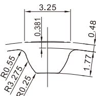
标准齿形
