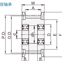
双轴承
