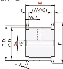
带轮形状:A型
