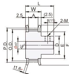
带轮形状:B型
