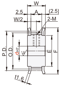
带轮形状:A型
