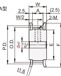
轴孔规格
