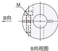
B向视图
