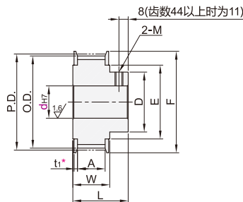
带轮形状:B型
