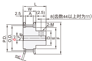
带轮形状:B型
