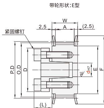
带轮形状:E型
