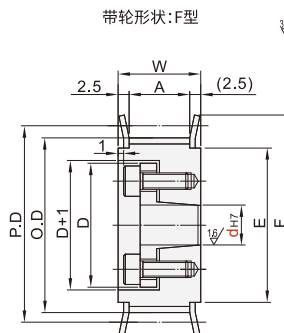
带轮形状:F型
