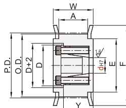
带轮形状:F型
