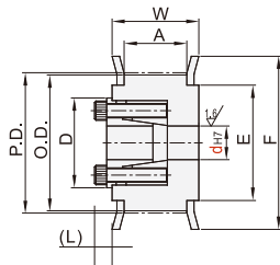
带轮形状:E型
