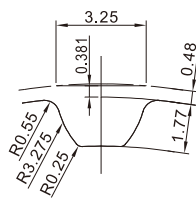
标准齿形
