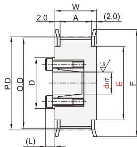
带轮形状:E型
