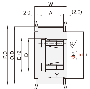
带轮形状:F型
