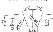
齿形(ISO标准齿条尺寸)
