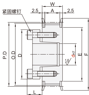
带轮形状:E型
