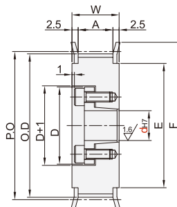
带轮形状:F型
