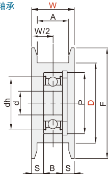
带法兰 单轴承
