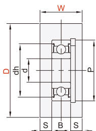
无法兰 单轴承
