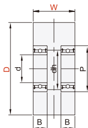
无法兰 双轴承
