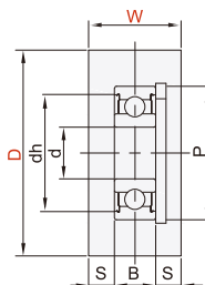
无法兰 单轴承
