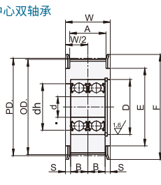
中心双轴承
