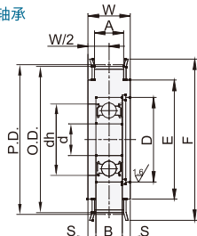
单轴承
